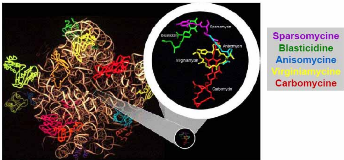
Figure 4 - L'enzyme qui catalyse la synthèse des protéines au sein de l'unité ribosomique 50 S est inhibée par une série d'antibiotiques qui se fixent d'une façon précise sur elle, positions qui ont été déterminées de façon exquise par les travaux des trois lauréats (études cristallographiques).
