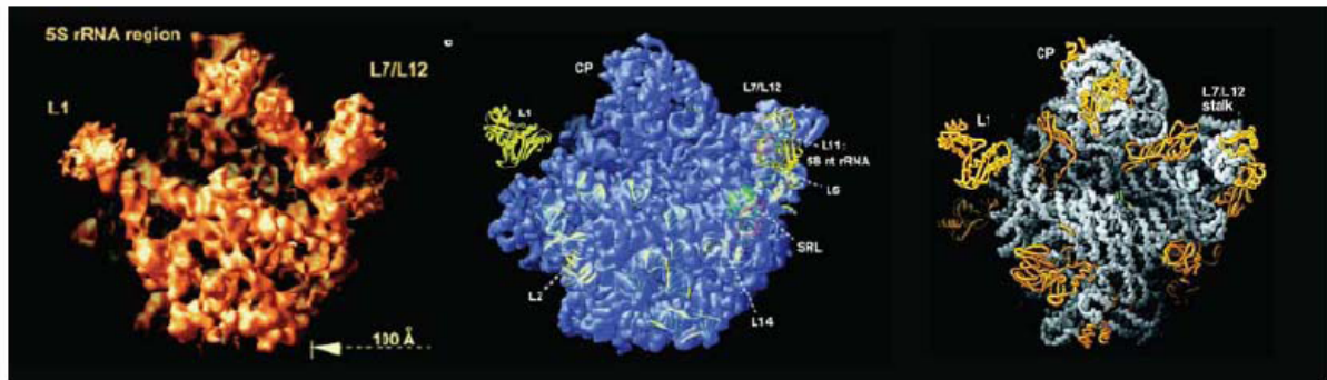
Figure 3 - La même unité 50 S vue avec une résolution de 0,9 nm (à gauche), de 0,5 nm (au centre) et de 0,1 nm (à droite). Le nm (nanomètre) est un milliardième de mètre. À droite les tresses bleuâtres sont de l'ARN ribosomique et les éléments jaunâtres sont des protéines intrinsèques de l'unité 50 S.
